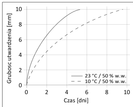
Wykres 1: Szybkość utwardzania Sikaflex®-228
