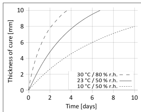
Wykres 1: Szybkość utwardzania Sikaflex®-263
