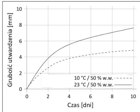
Wykres 1: Szybkość utwardzania Sikaflex®-529 Evolution
