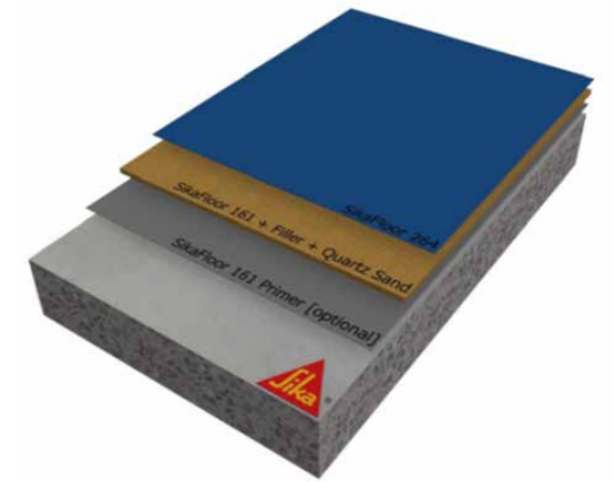
SYSTEM SIKAFLOOR®-ES14 DLA POZIOMÓW POŚREDNICH
