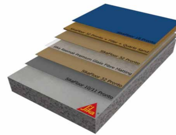
SYSTEM SIKAFLOOR®-RB58 DLA KONDYGNACJI DACHOWEJ
