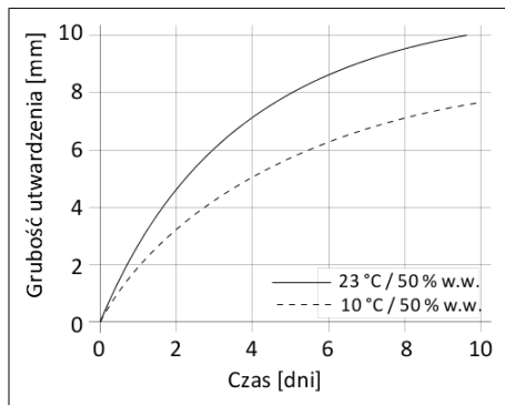
Wykres 1: Szybkość utwardzania Sikaflex®-515
