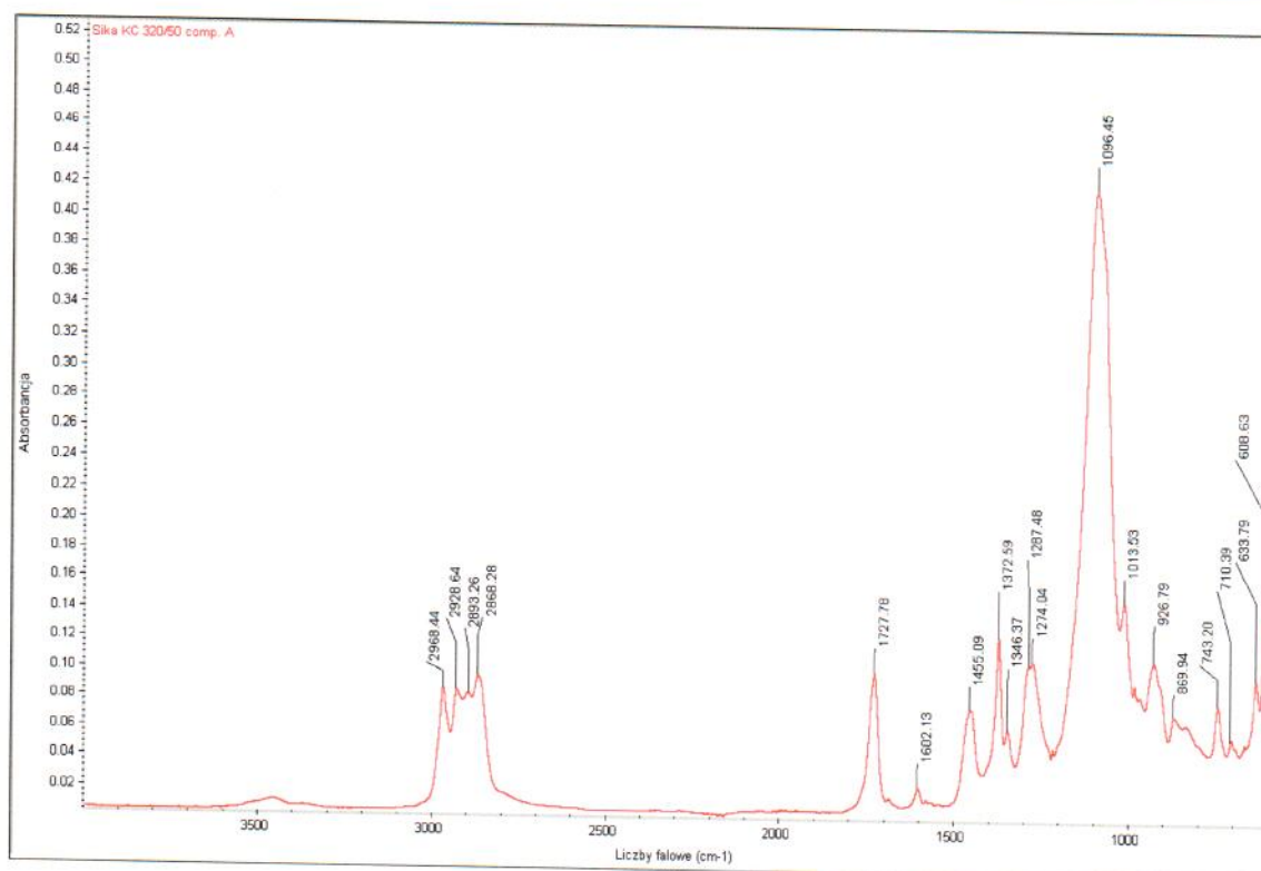
Rysunek 11 – Widmo w podczerwieni (analiza FTIR) składnika A masy Icosit® KC 320/50
