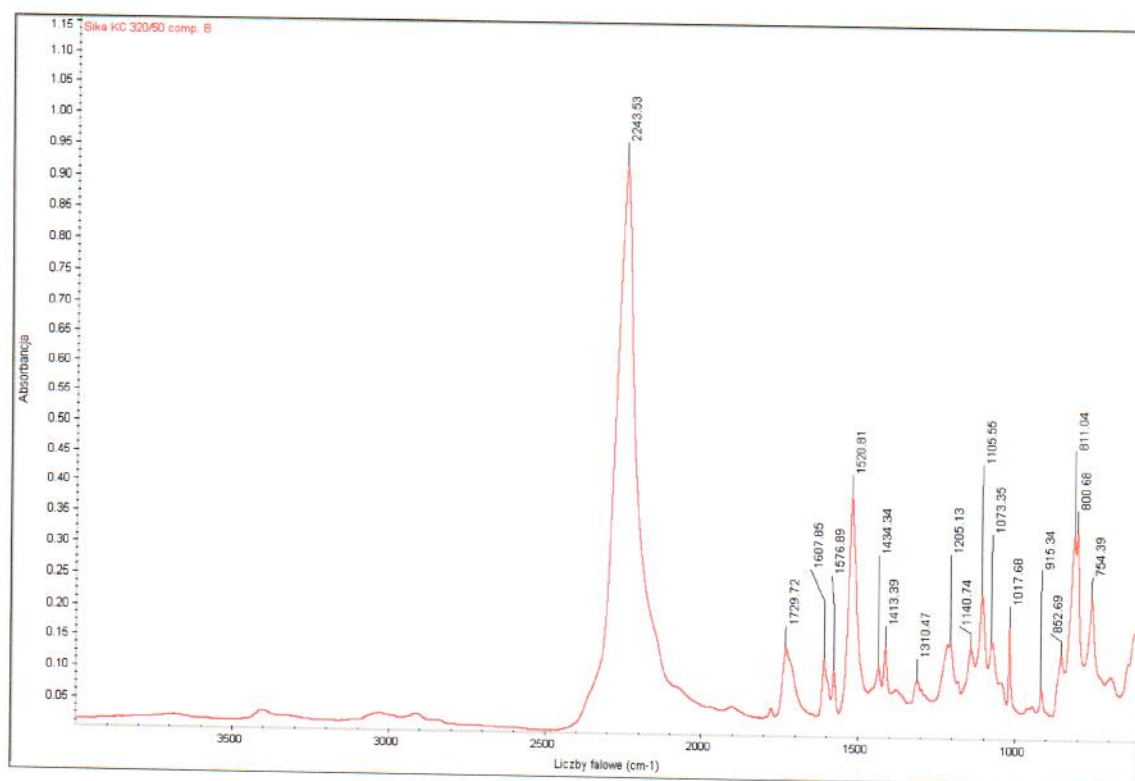
Rysunek 12 – Widmo w podczerwieni (analiza FTIR) składnika B masy Icosit® KC 320/50
