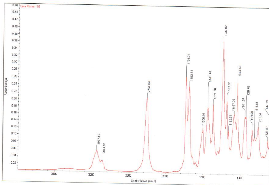
Rysunek 2 – Widmo w podczerwieni (analiza FTIR) środka gruntującego Sika® Primer-115
