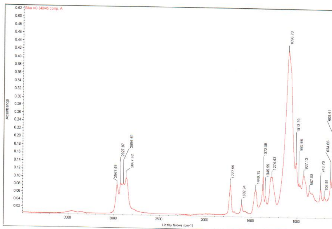
Rysunek 5 – Widmo w podczerwieni (analiza FTIR) składnika A masy Icosit® KC 340/45
