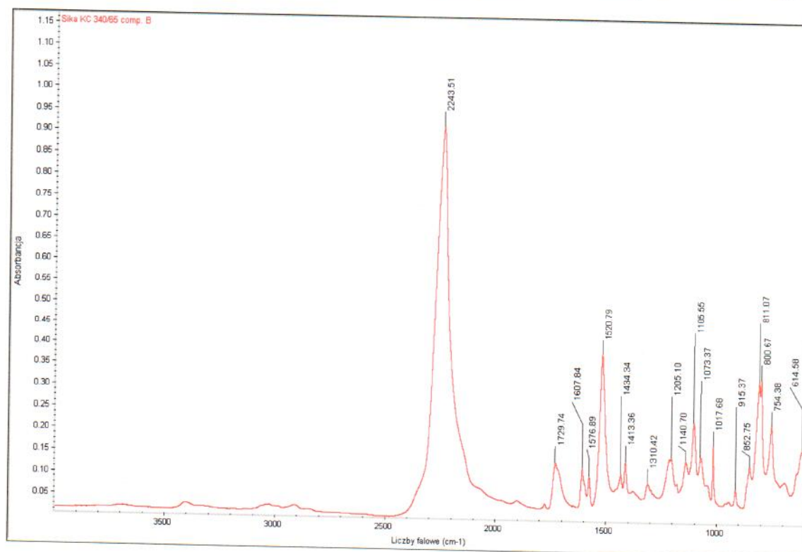
Rysunek 8 – Widmo w podczerwieni (analiza FTIR) składnika B masy Icosit® KC 340/65
