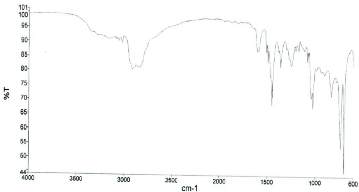
Rysunek 16 – Widmo w podczerwieni (analiza FTIR) składnika B żywicy Sikadur®-53
