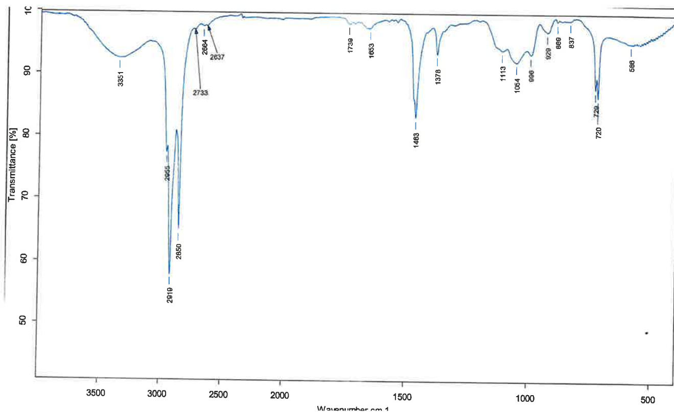
Rysunek Z.1 – Widmo w podczerwieni Sika® Rugasol-33 OVZ.
