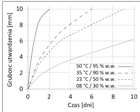
Wykres 1: Szybkość utwardzania Sikasil® SG-20
