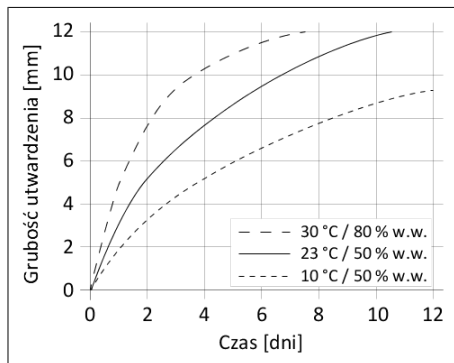
Wykres 1: Szybkość utwardzania Sikaflex®-821 FR
