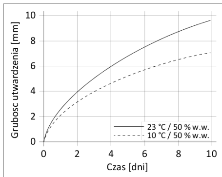
Wykres 1: Szybkość utwardzania Sikaflex®-508
