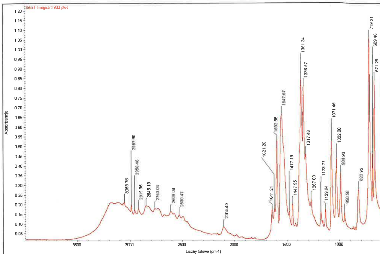
Rysunek 1– Widmo w podczerwieni (analiza FTIR) wyrobu Sika® FerroGard®-903 Plus
