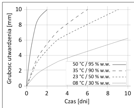
Wykres 1: Szybkość utwardzania Sikasil® WT-40
