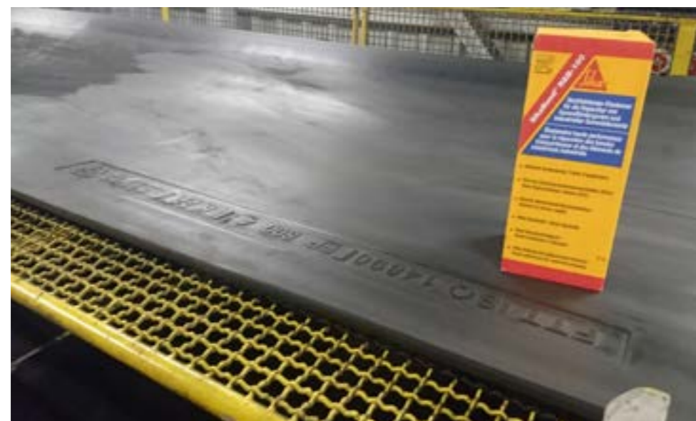
Pas transmisyjny przed naprawą. Widoczny stempel po stronie roboczej
