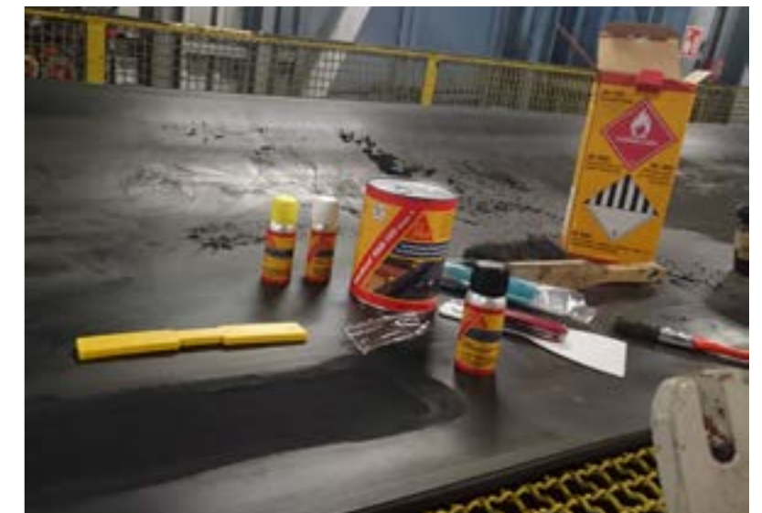
Powierzchnia pasa przygotowana do nakładania Sika Bond R&B 100
