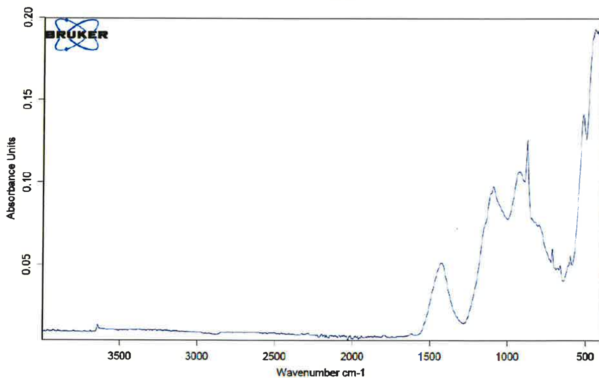
Rys. Z-1 Analiza w podczerwieni materiału Sika MonoTop®-910 N / Sika MonoTop®-2001 Bond & Protect.
