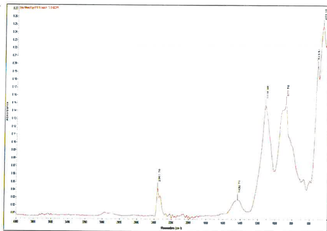
Rys. Z-1 Analiza w podczerwieni materiału Sika MonoTop®-910 N / Sika MonoTop®-2001 Bond & Protect.
