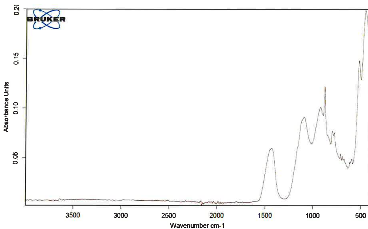
Rys. Z-4 Analiza w podczerwieni materiału Sika MonoTop®-4012.
